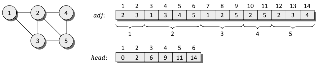
Hình 5-8. Dùng mảng biểu diễn danh sách kề
